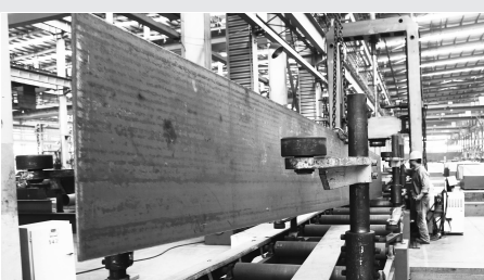
小小吊板支架用大▲组立焊接笔直“一条线”▶
